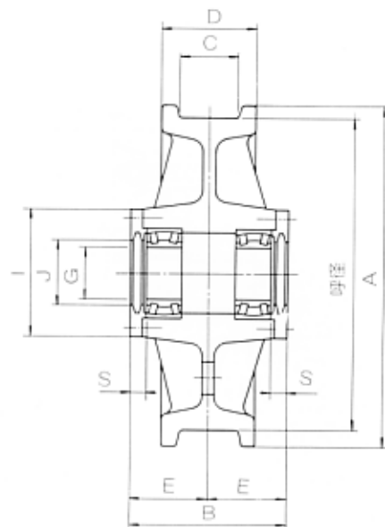
従動車C (車輪踏面巾C-125)
