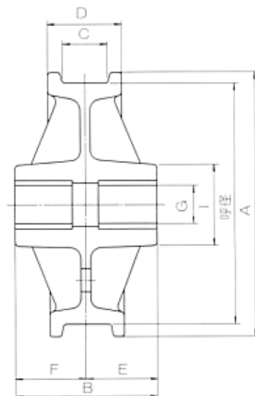
従動車A (車輪踏面巾C-63)
