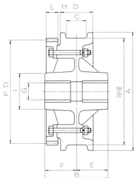
駆動車A (車輪踏面巾C-63)
