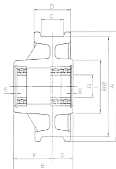
従動車A (車輪踏面巾C-60)
