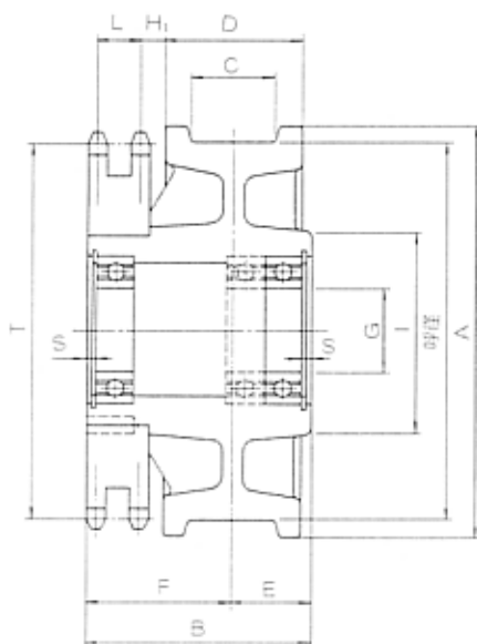
従動車A (車輪踏面巾C-60)
