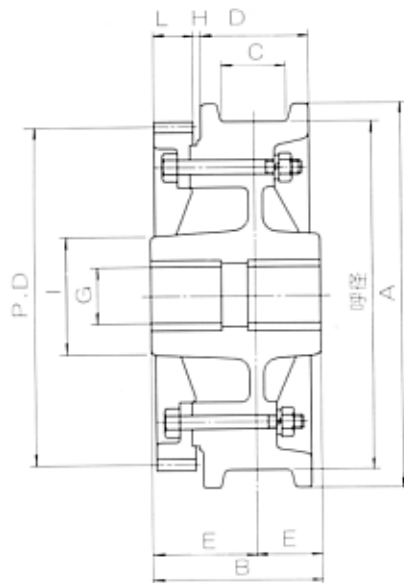
駆動車A (車輪踏面巾C-60)
