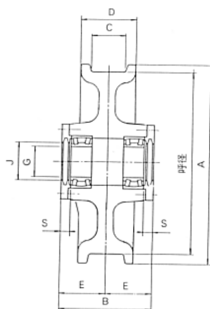
従動車 C (車輪踏面巾 C - 125)
