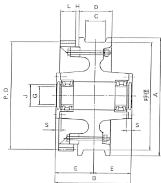
駆動車 C (車輪踏面巾 C - 125)
